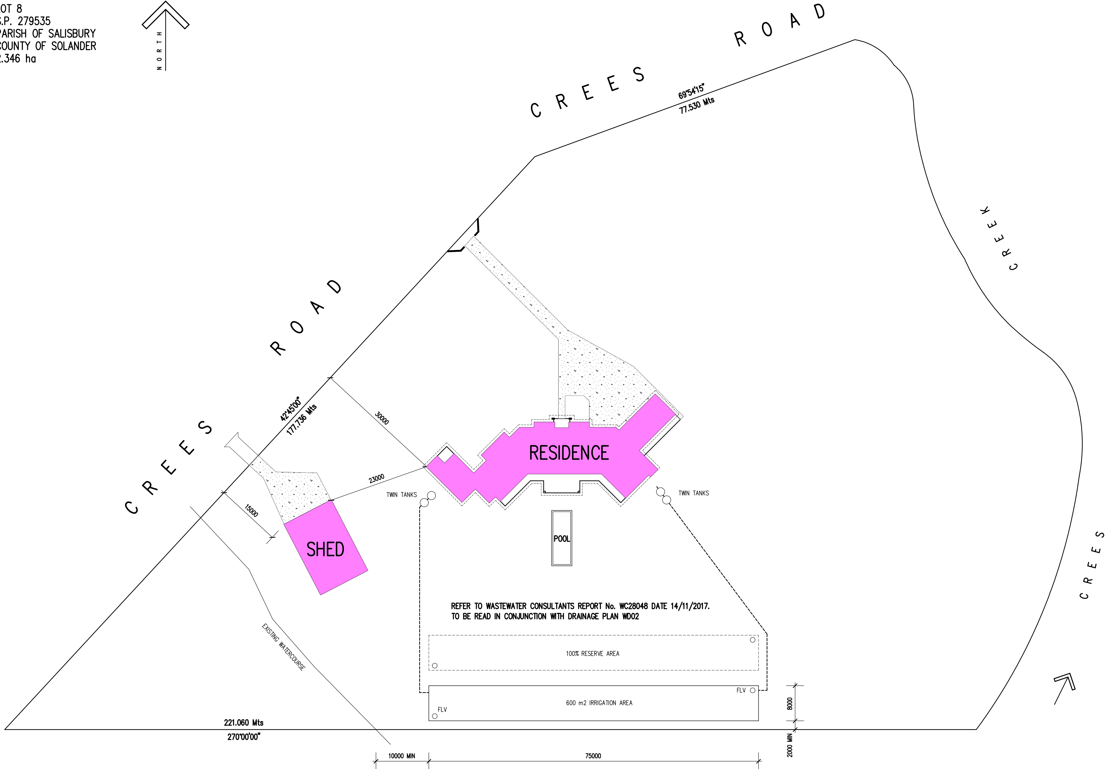
SITE PLAN 1:500
