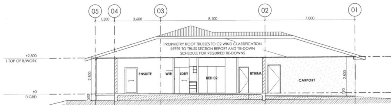
Section 02 1:100
