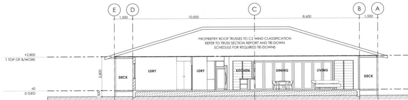
Section 01 1:100
