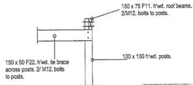
DETAIL A. 1:20.
