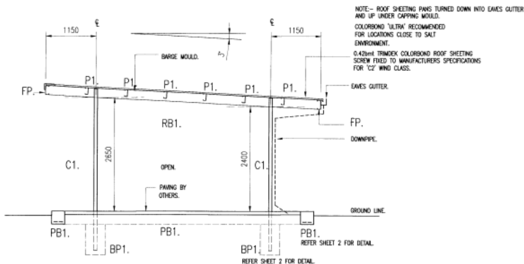
SECTION A-A. SCALE :- 1:50 2
