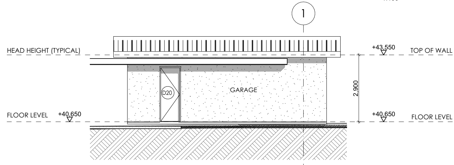
E7 ELEVATION 1:100
