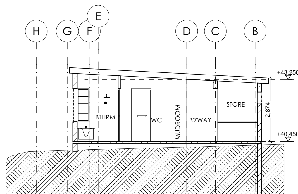
SECTION S6 1:100
