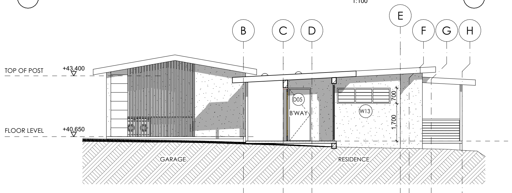
E8 ELEVATION 1:100
