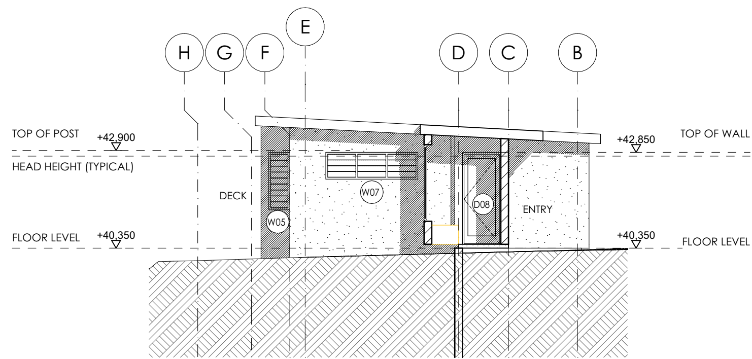
E6 ELEVATION 1:100
