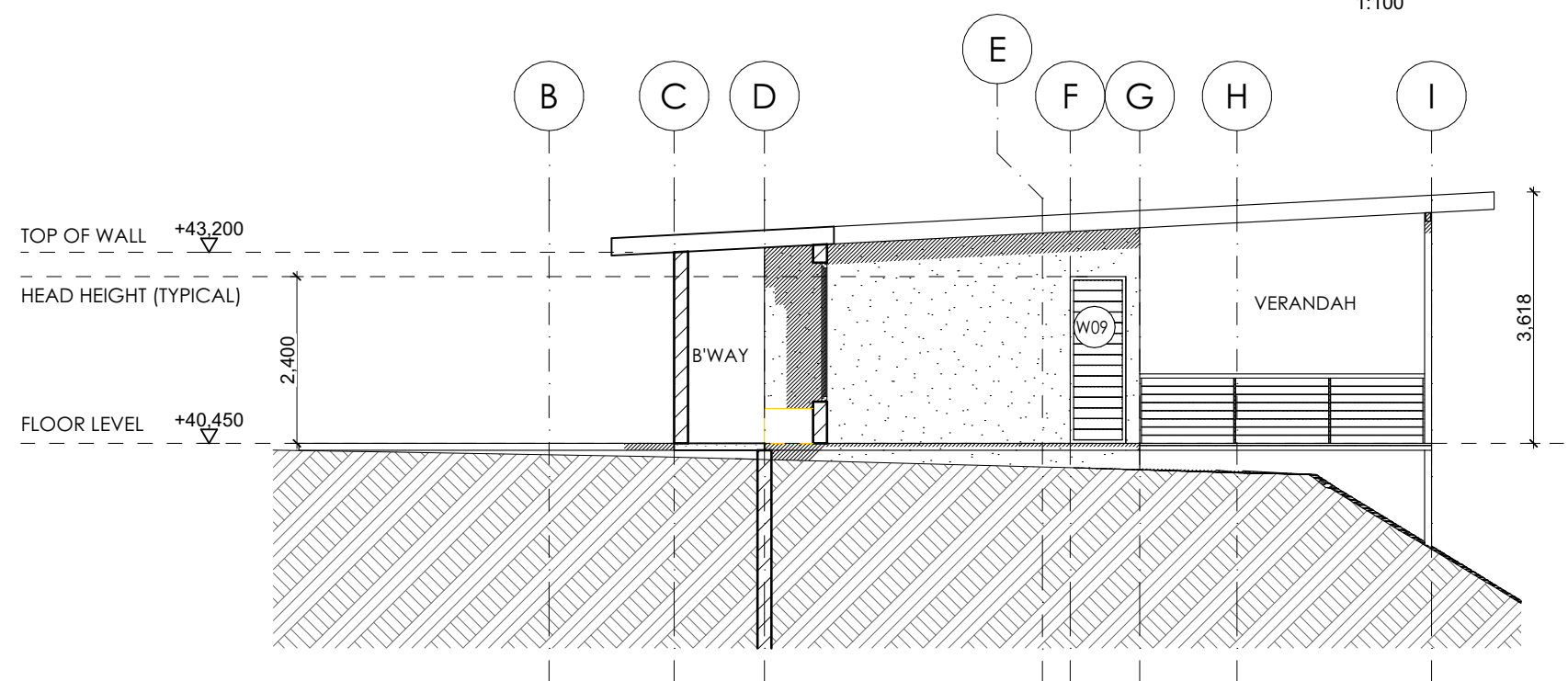
E7 ELEVATION 1:100
