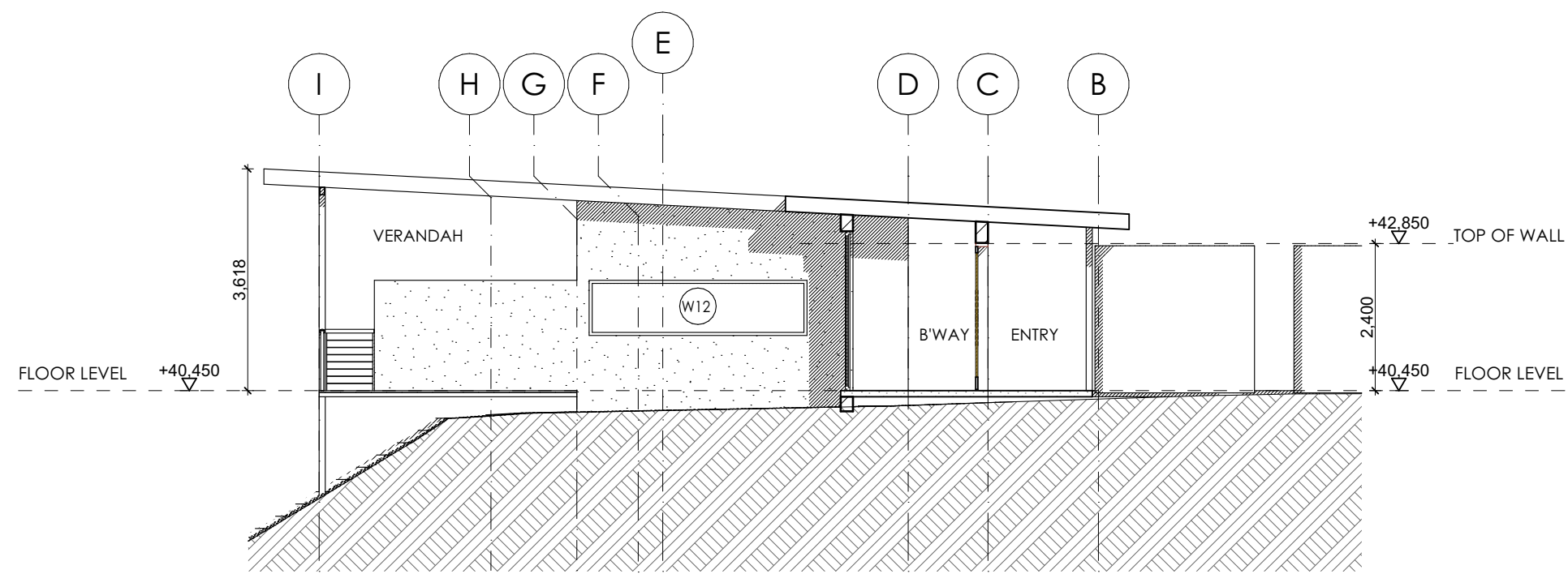
E5 ELEVATION 1:100
