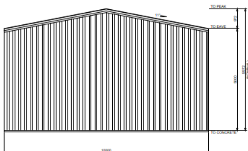
4 ENDWALL EXTERIOR ELEVATION SCALE: 1 = 100
