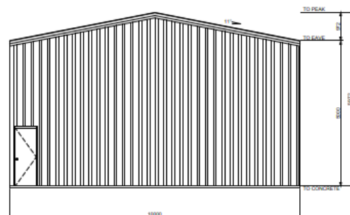
3 ENDWALL EXTERIOR ELEVATION SCALE: 1 = 100
