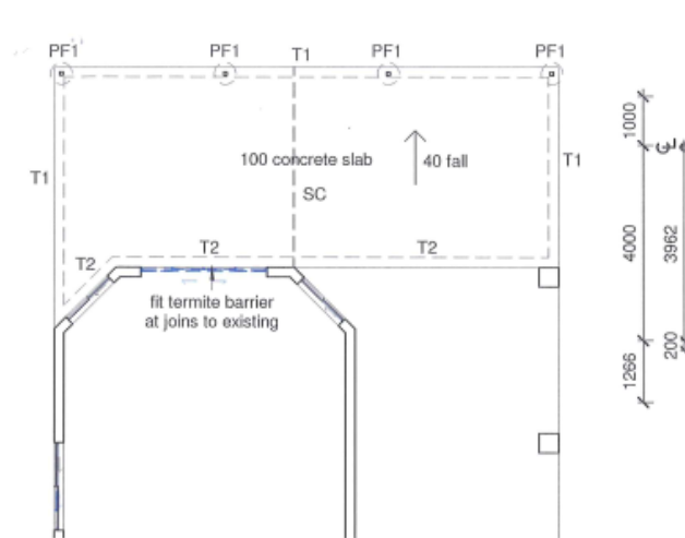
1 Foundation Plan 1 : 100
