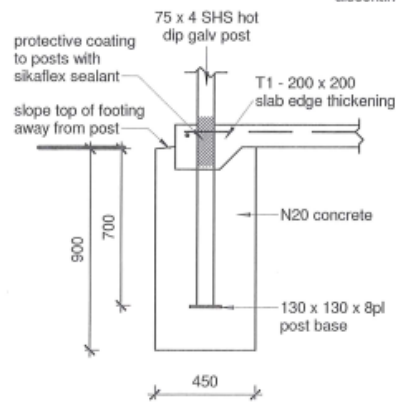
A PF1 Footing 1 : 20
