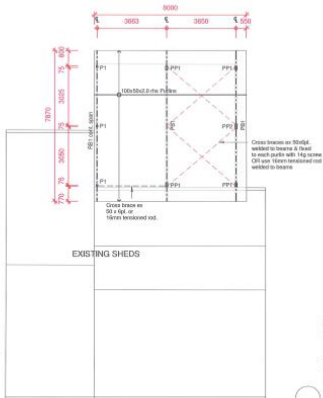
① Roof Frame Plan 1 : 100
