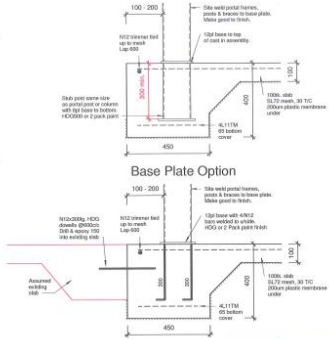
2 Edge beam 1 : 10
