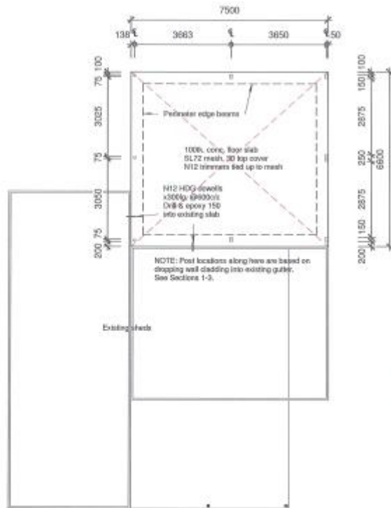
1 Foundation Plan 1 : 100
