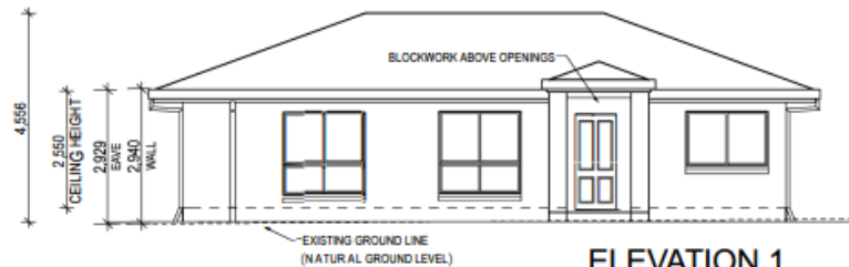
ELEVATION 1
