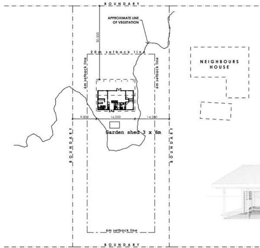
SITE PLAN 1:500
