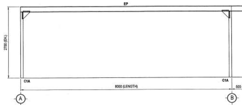
ELEVATION FRAMING GL.B SCALE 1:50
