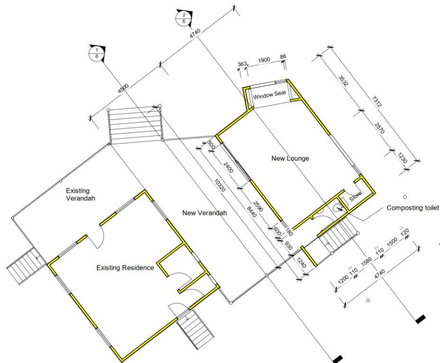
1 FLOOR PLAN 1 : 100
