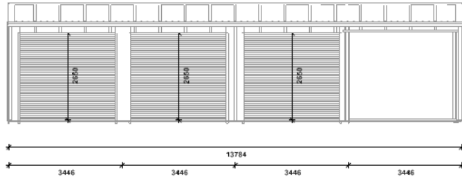
ELEVATION 1
