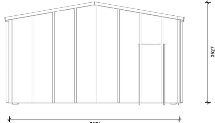
ELEVATION 2
