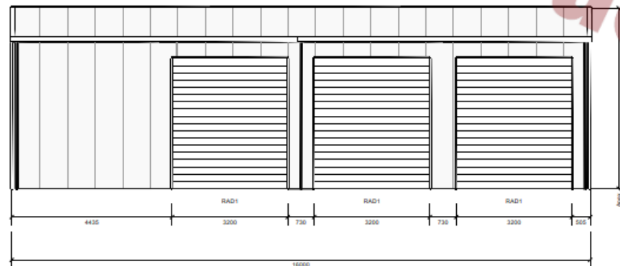
RIGHT ELEVATION
