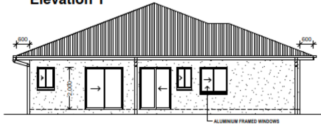
Elevation 2
