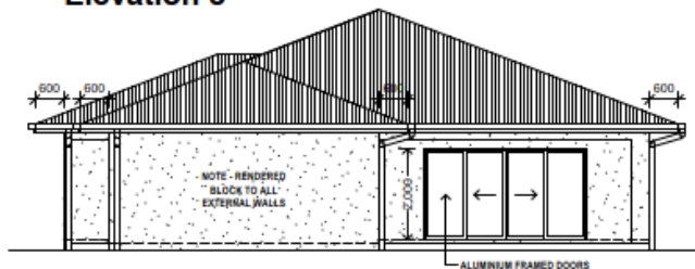
Elevation 4
