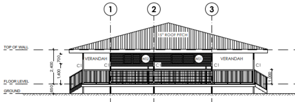
ELEVATION 02 1:100
