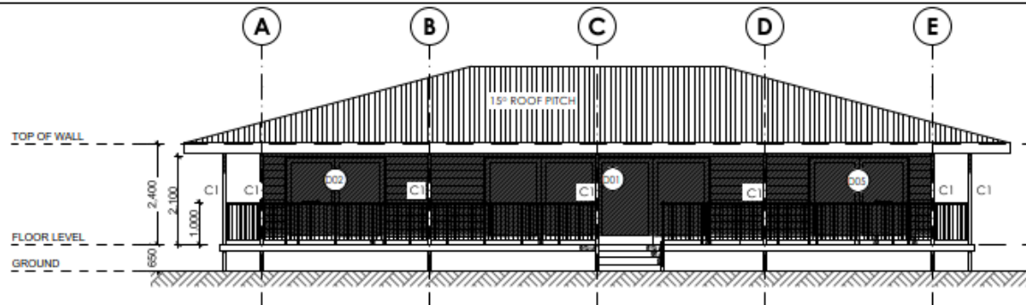
ELEVATION 01 1:100
