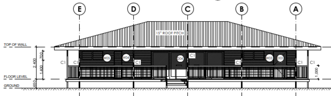
ELEVATION 03 1:100
