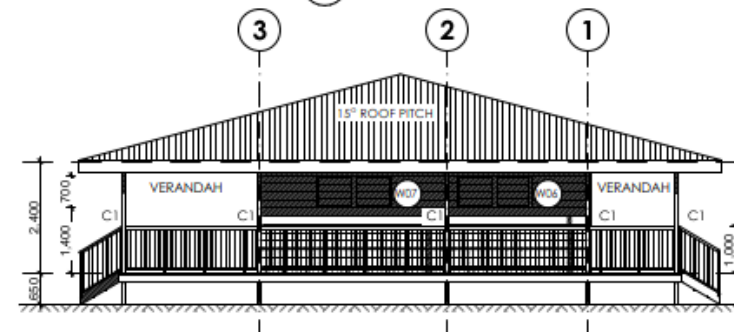
ELEVATION 04 1:100
