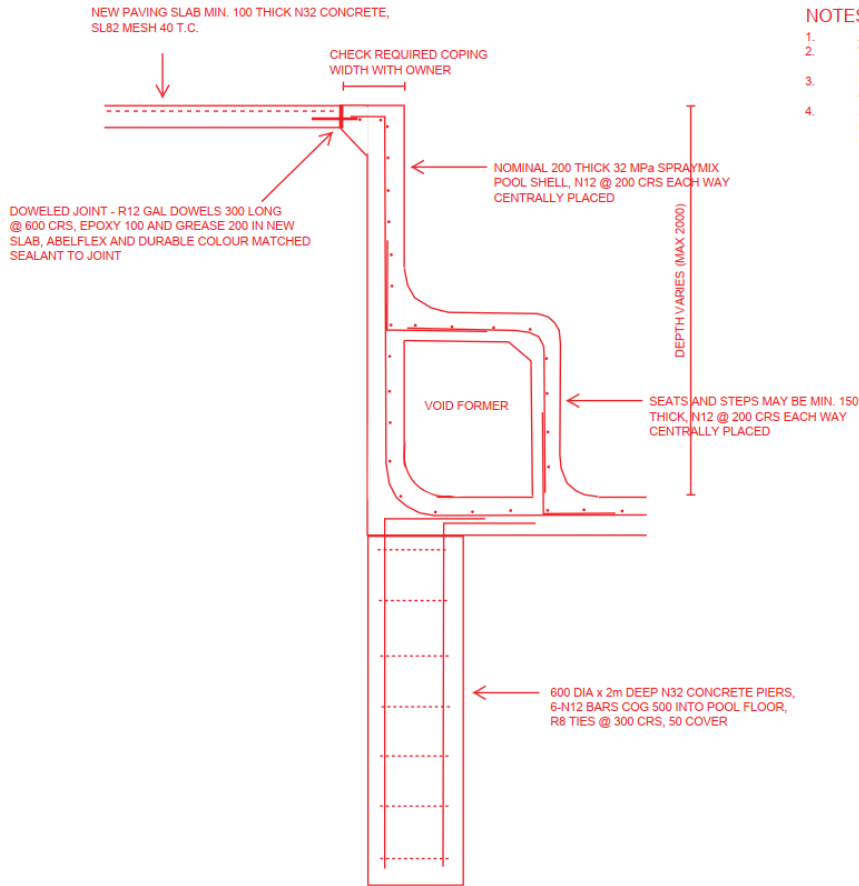
TYP. POOL SECTION N.T.S.
