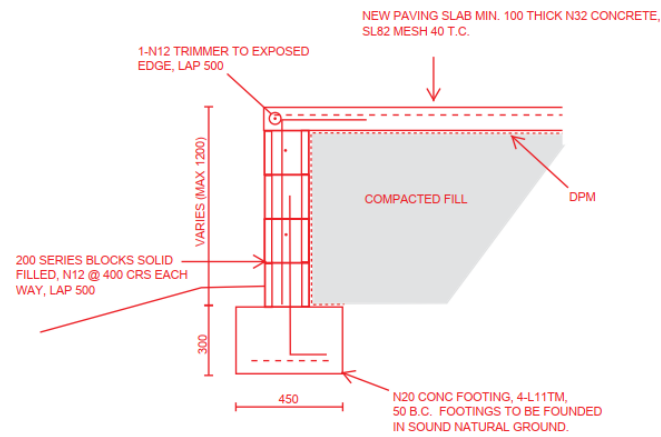
STRIP FOOTING N.T.S.
